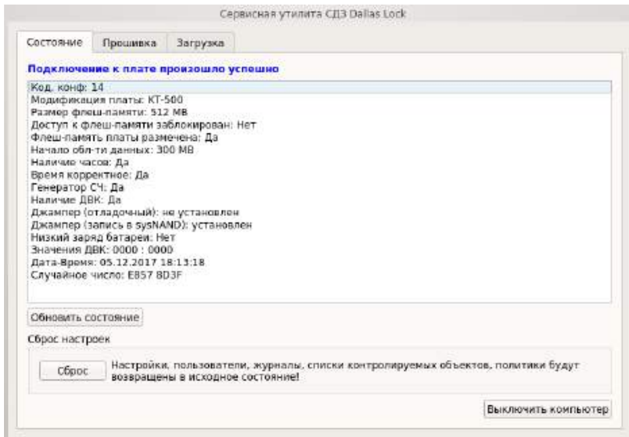
Рисунок 58 – Сервисная утилита
