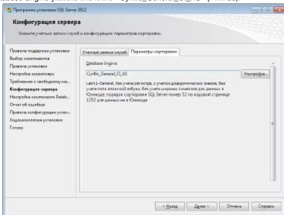
Рис. 28. Параметры сортировки
