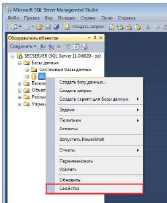
Рис. 38 – Обозреватель объектов
