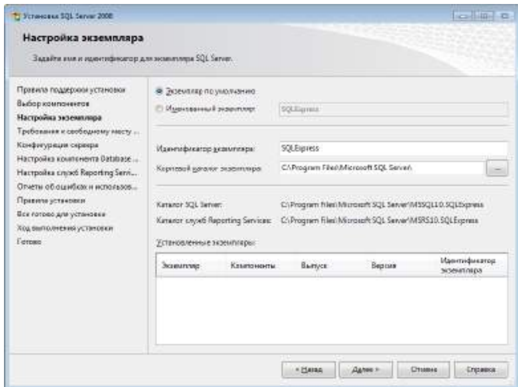
Рис. 10. Настройка экземпляра
