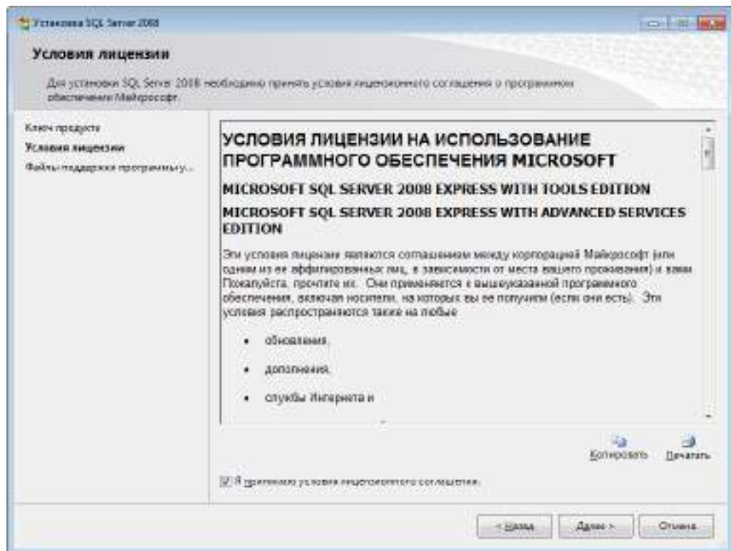
Рис. 6. Условия лицензии
