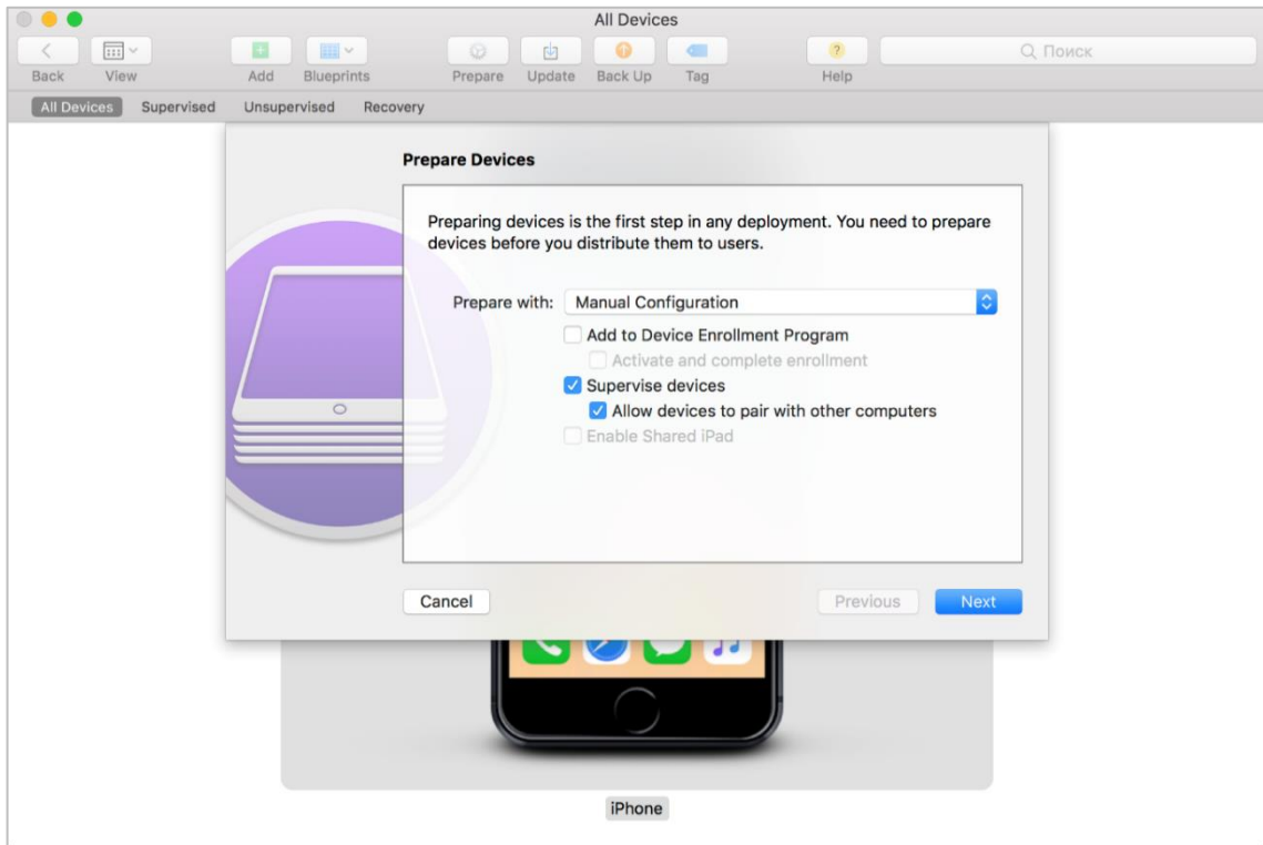
Рисунок А.2 – Выбор режима подготовки устройства
