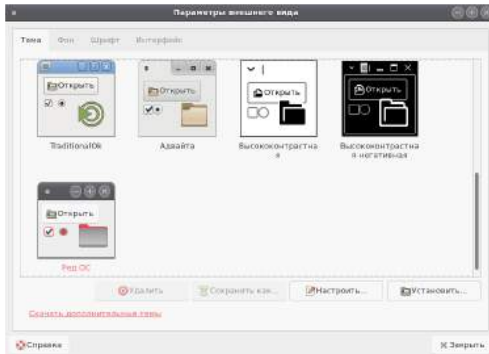
Рисунок 3.16 – Утилита «Параметры внешнего вида», вкладка «Тема»
