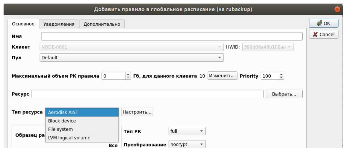
Рис. 7. Выбор типа ресурса для правила резервного копирования.
