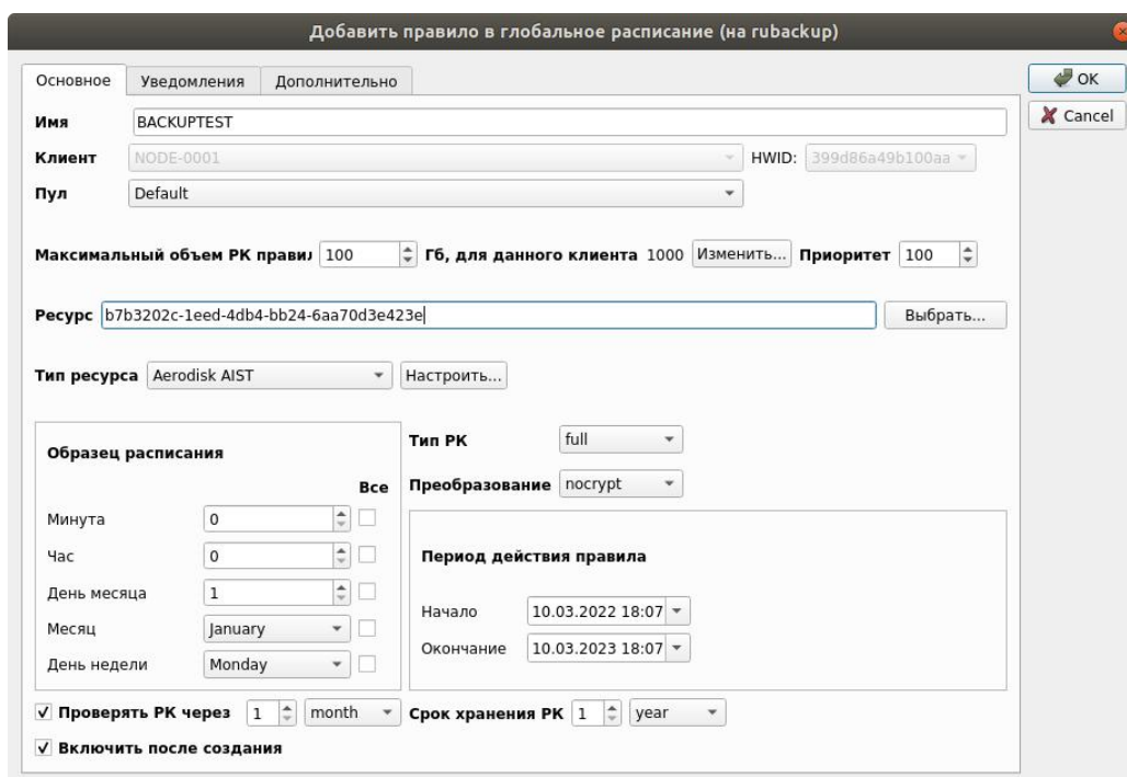
Рис. 9. Настройки правила резервного копирования.
