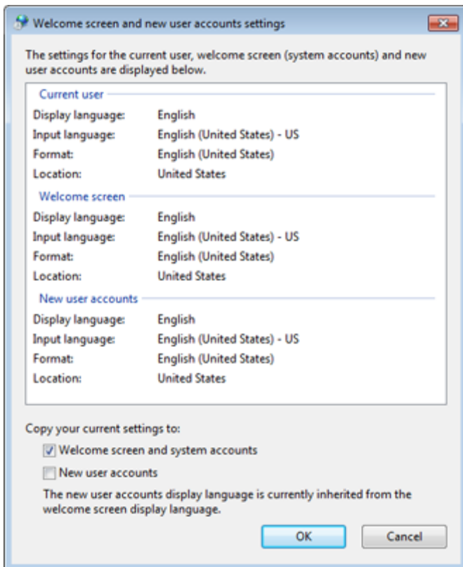
Рисунок 38. Копирование параметров
