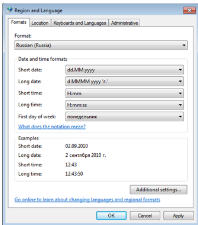
Рисунок 39. Настройка форматов
