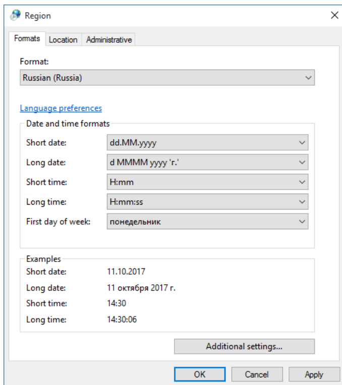
Рисунок 44. Настройка форматов
