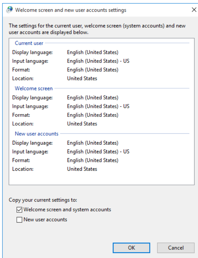
Рисунок 43. Копирование параметров
