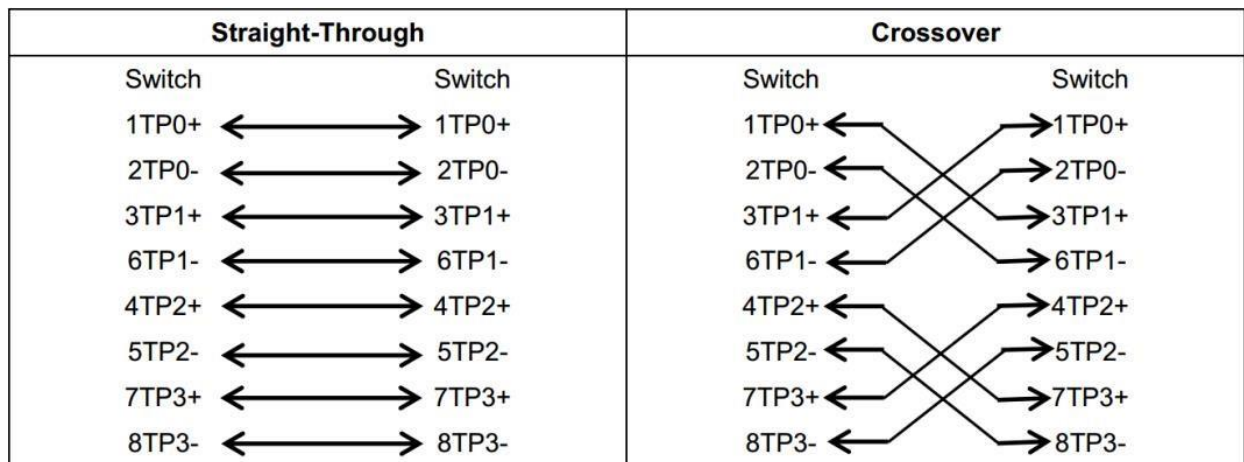
Рисунок 21. Четыре витых пары для порта 1000 BASE-T
