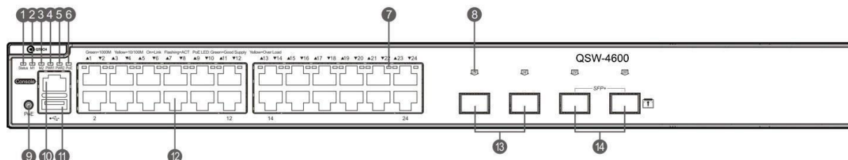
Рисунок 5. Передняя панель QSW-4600-28TX-POE
