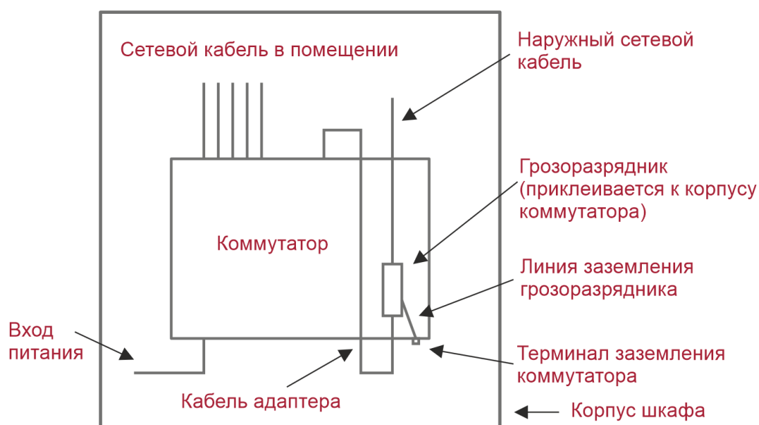
Рисунок 26. Схематическая диаграмма грозозащитника на Ethernet-порте
