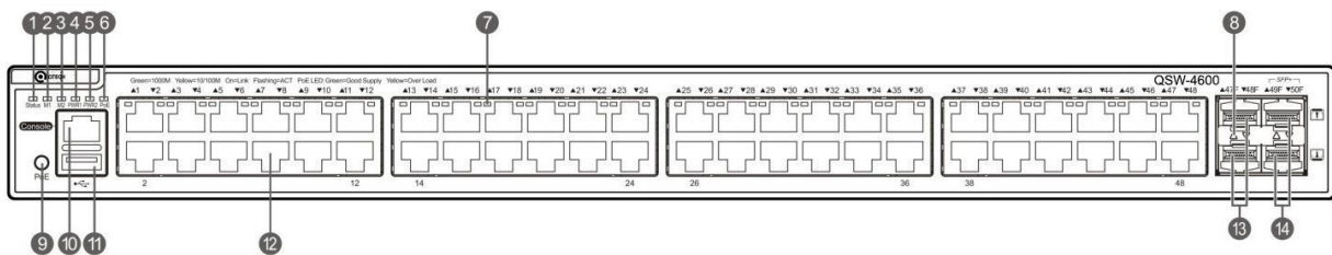
Рисунок 8. Передняя панель QSW-4600-52TX-POE
