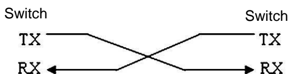
Рисунок 24. Подключение по волоконной оптике
