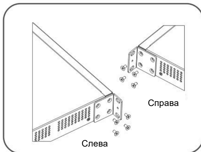
Рисунок 12. Присоединение крепежных кронштейнов к коммутатору
