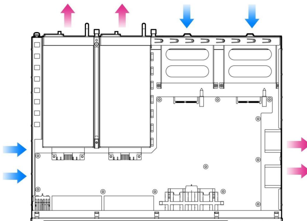
Рисунок 7. Схема вентиляции системы охлаждения.
