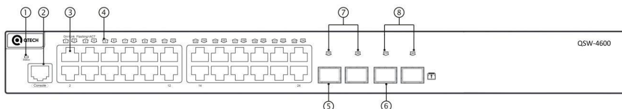
Рисунок 1. Передняя панель QSW-4600-28TX
