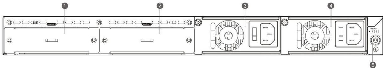
Рисунок 9. Задняя панель QSW-4600-52TX-POE
