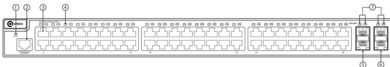
Рисунок 3. Передняя панель QSW-4600-52TX
