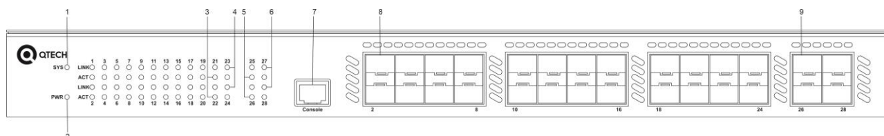
Рисунок 1-19 Передняя панель QSW-3310-28F-AC-DC
