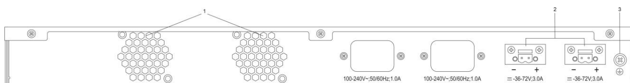
Рисунок 1-22 Задняя панель QSW-3310-28F-DC-DC
