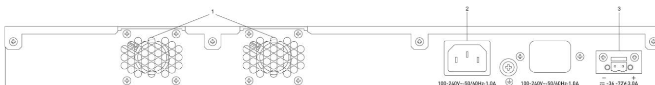
Рисунок 1-20 Задняя панель QSW-3310-28F-AC-DC
