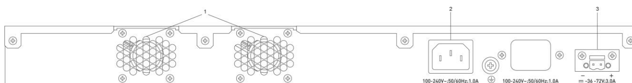
Рисунок 1-8 Задняя панель QSW-3310-28TX-AC-DC
