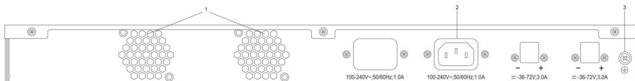
Рисунок 1-2 Задняя панель QSW-3310-28TX-AC
