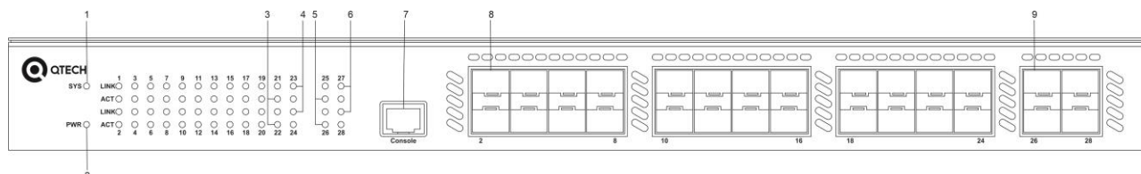
Рисунок 1-13 Передняя панель QSW-3310-28F-AC
