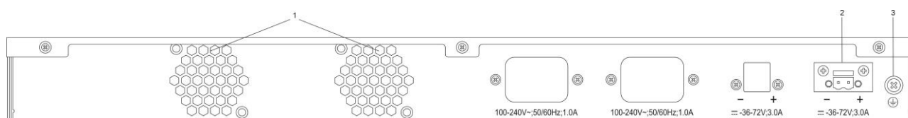
Рисунок 1-4 Задняя панель QSW-3310-28TX-DC
