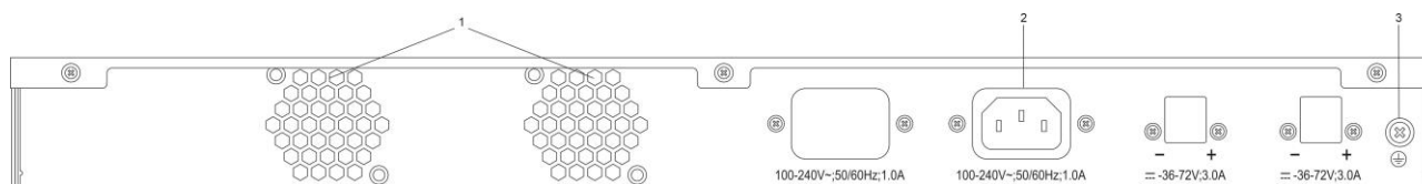
Рисунок 1-14 Задняя панель QSW-3310-28F-AC
