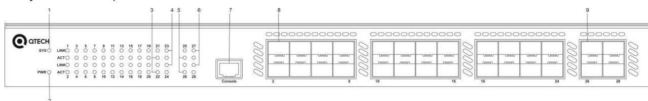
Рисунок 1-15 Передняя панель QSW-3310-28F-DC
