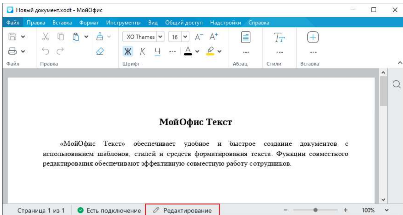
Рисунок 260 – Уровень доступа
