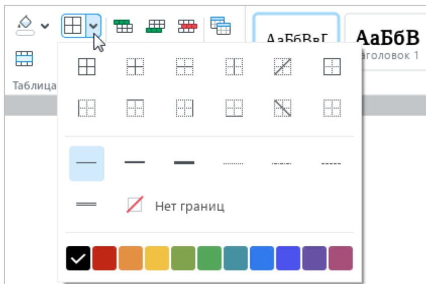
Рисунок 51 – Настройка границ
