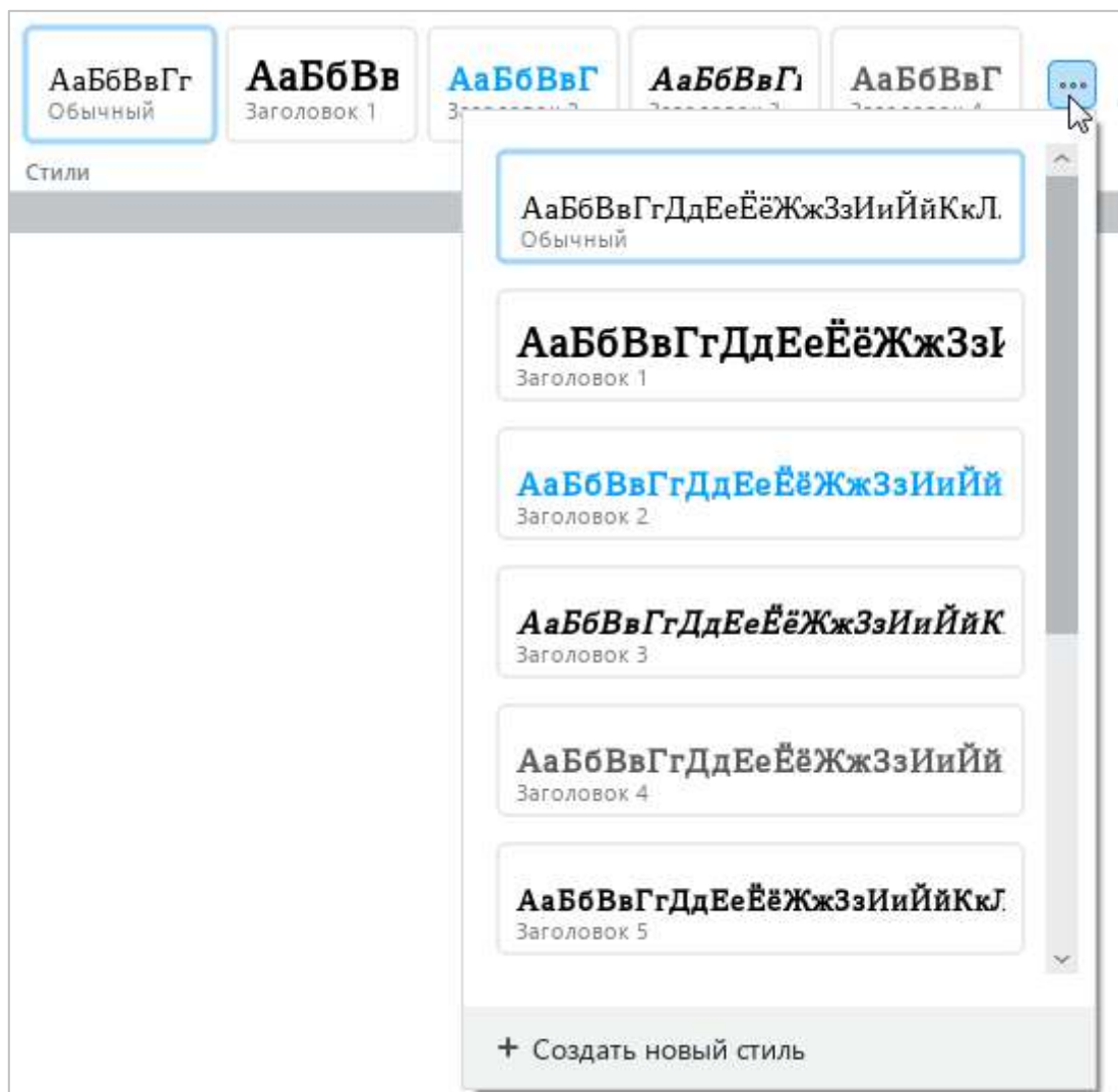
Рисунок 212 – Список стилей
