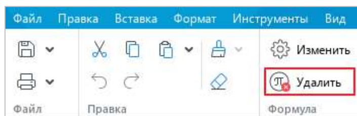
Рисунок 200 – Кнопка Удалить
