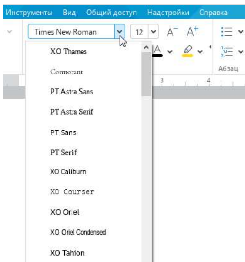
Рисунок 125 – Список шрифтов
