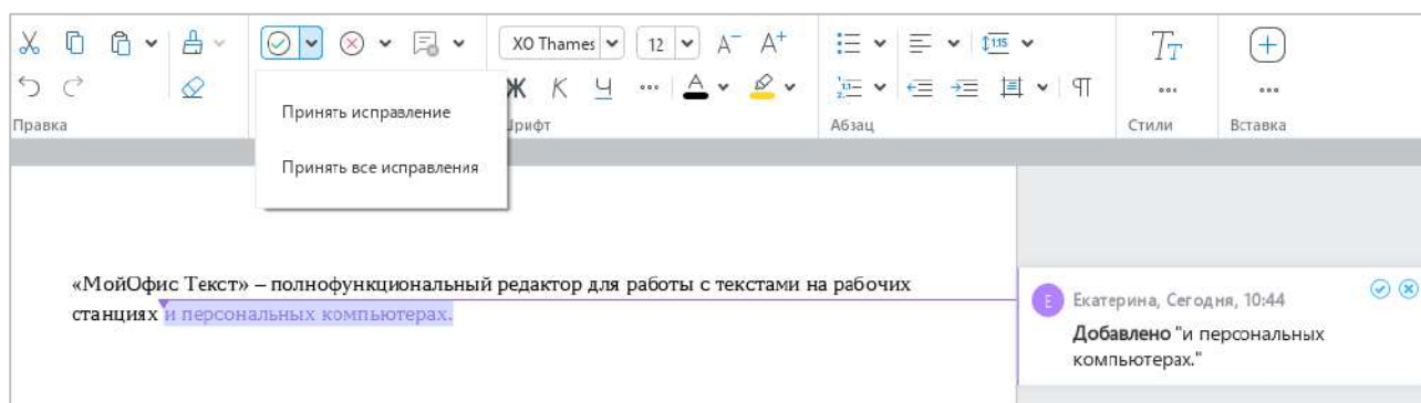
Рисунок 238 – Принятие исправлений
