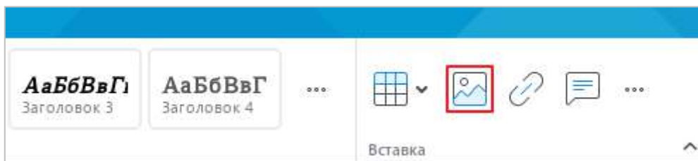
Рисунок 168 – Кнопка Изображение
