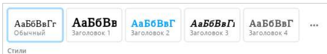
Рисунок 45 – Раздел Стили
