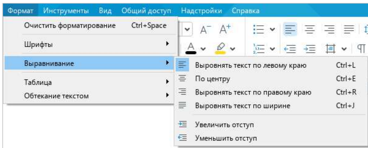
Рисунок 9 – Подменю Выравнивание
