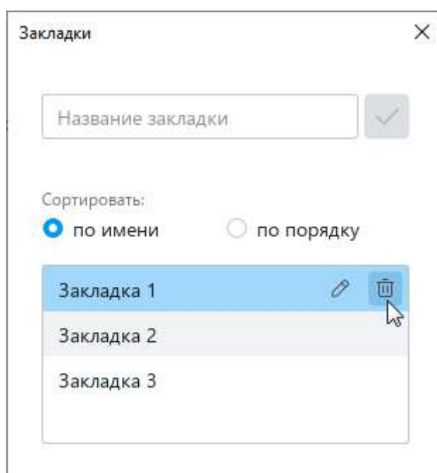
Рисунок 114 – Удаление закладки
