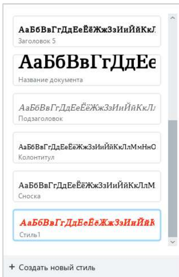
Рисунок 123 – Пользовательский стиль
