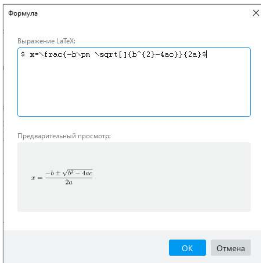
Рисунок 197 – Окно Формула
