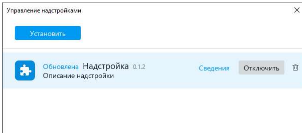
Рисунок 308 – Надстройка обновлена
