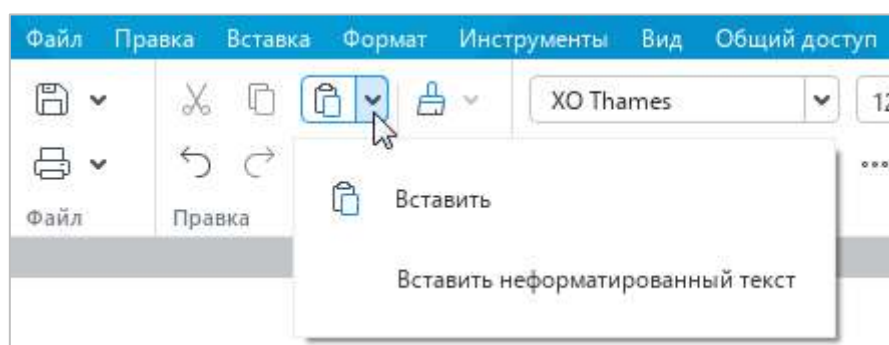
Рисунок 171 – Кнопка Вставить
