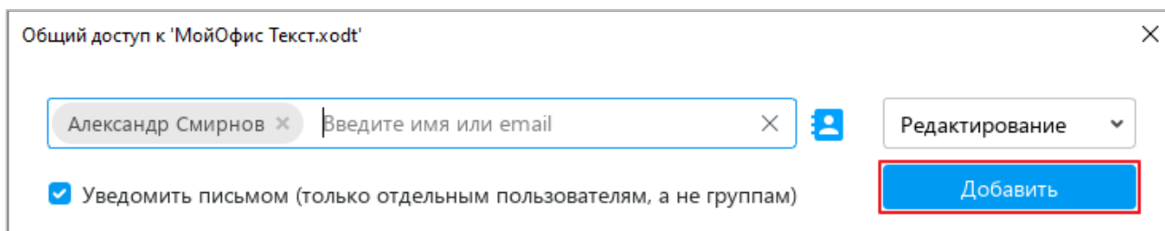
Рисунок 273 – Кнопка Добавить
