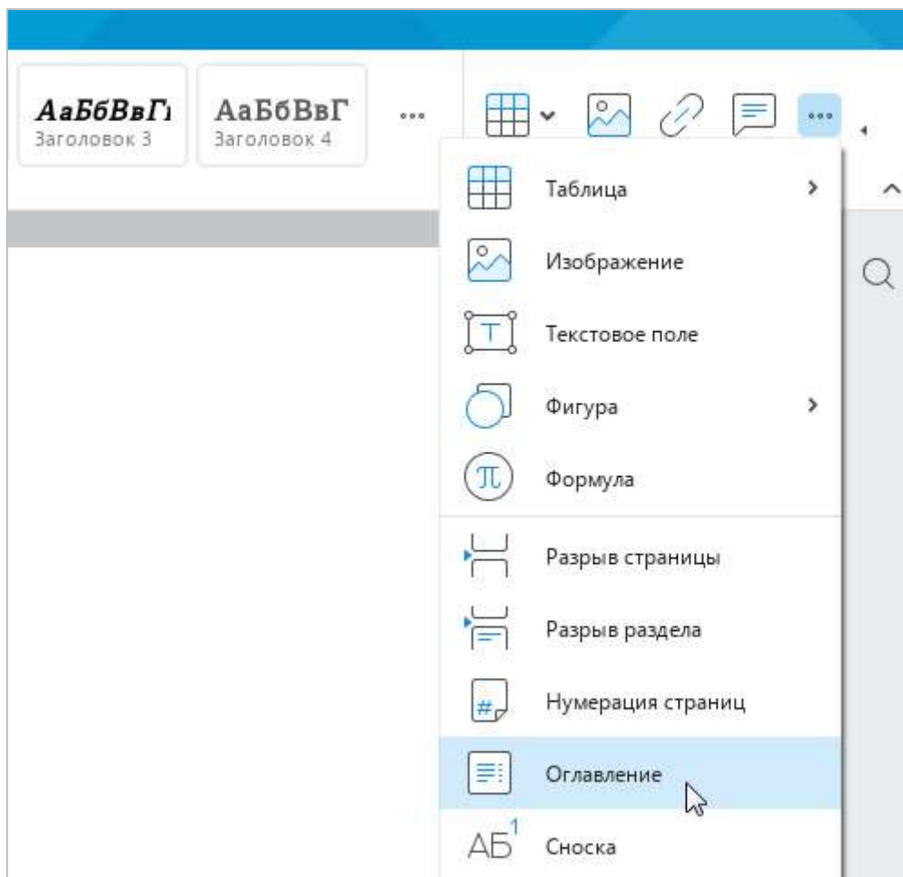
Рисунок 214 – Панель вставки
