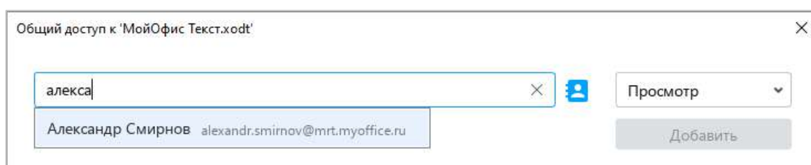
Рисунок 271 – Поиск пользователя
