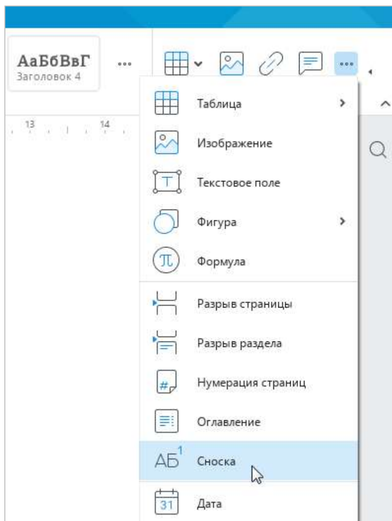
Рисунок 101 – Панель вставки
