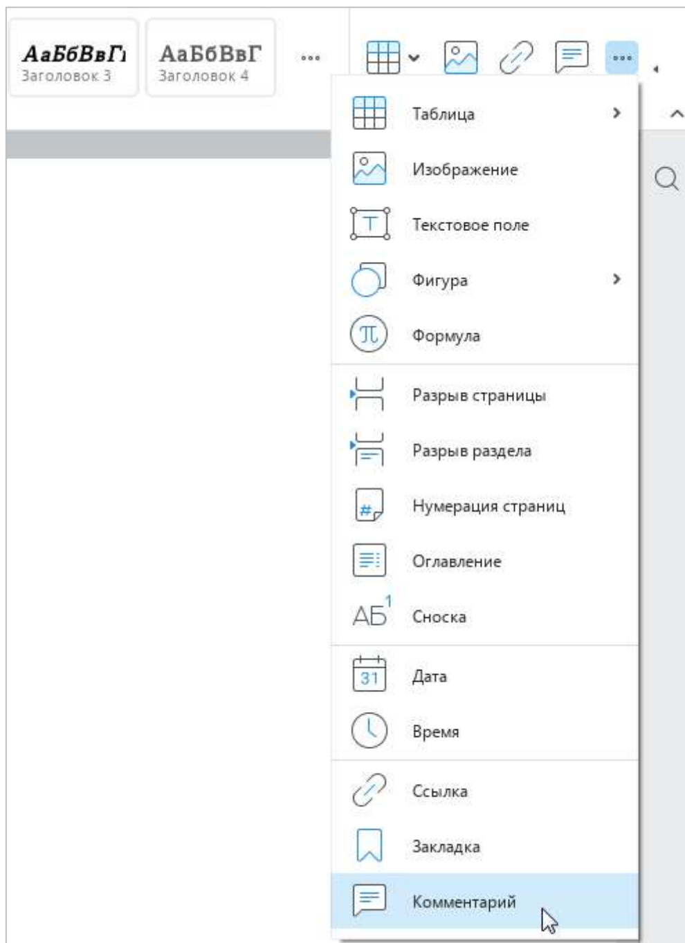
Рисунок 246 – Панель вставки
