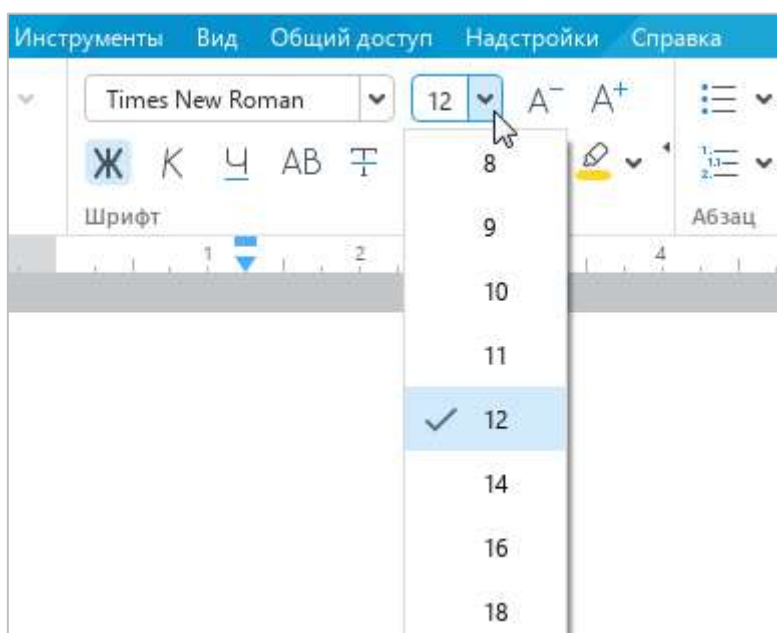
Рисунок 126 – Размер шрифта
