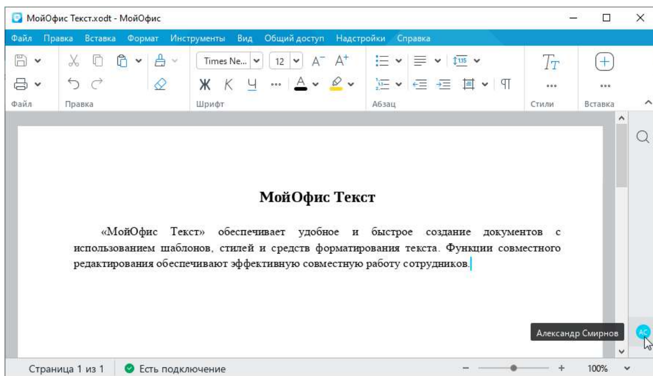
Рисунок 255 – Совместное редактирование
