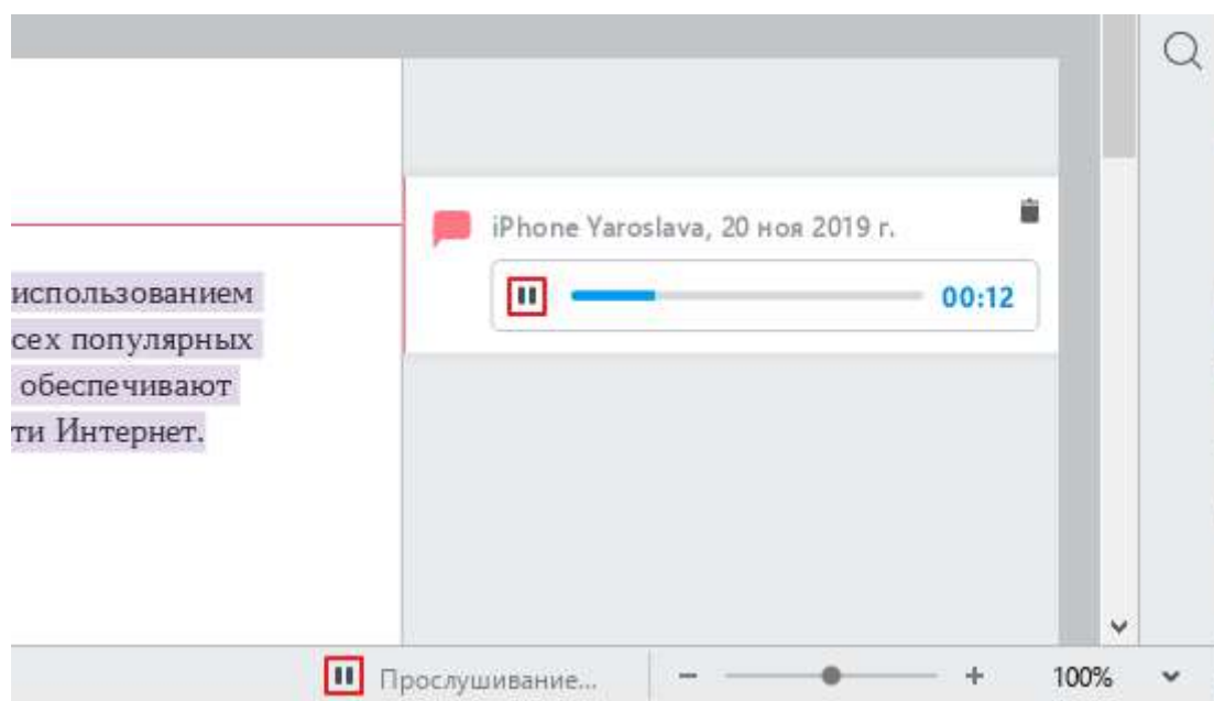
Рисунок 250 – Прослушивание аудиокomentarия
