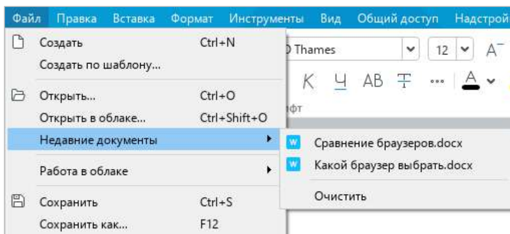
Рисунок 68 – Недавние документы
