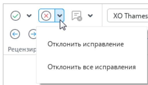
Рисунок 59 – Отклонение исправлений
