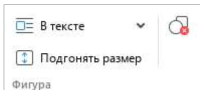
Рисунок 54 – Раздел Фигура
