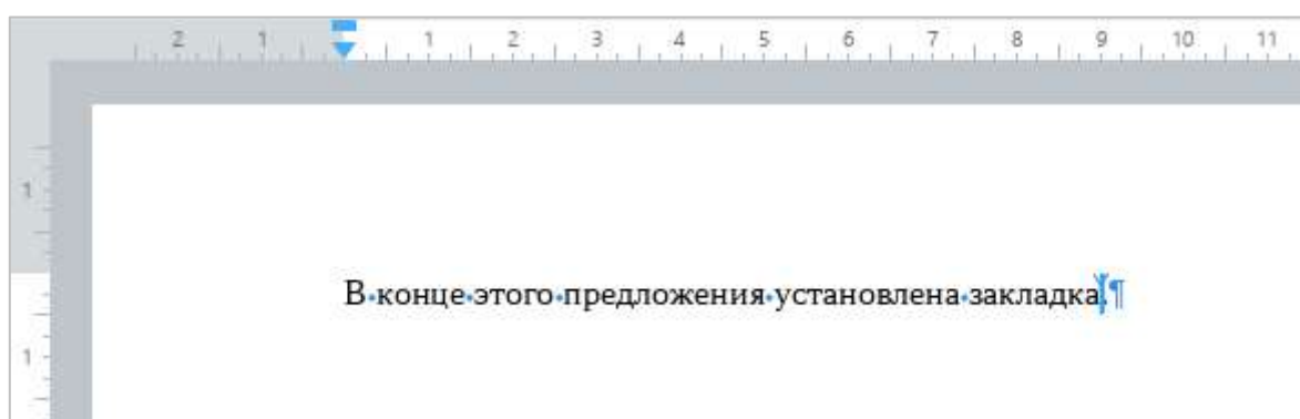
Рисунок 111 – Отображение закладки
