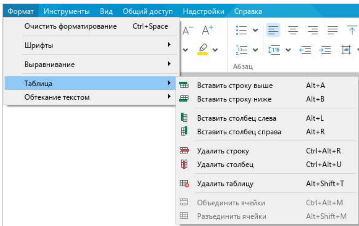
Рисунок 10 – Подменю Таблица
