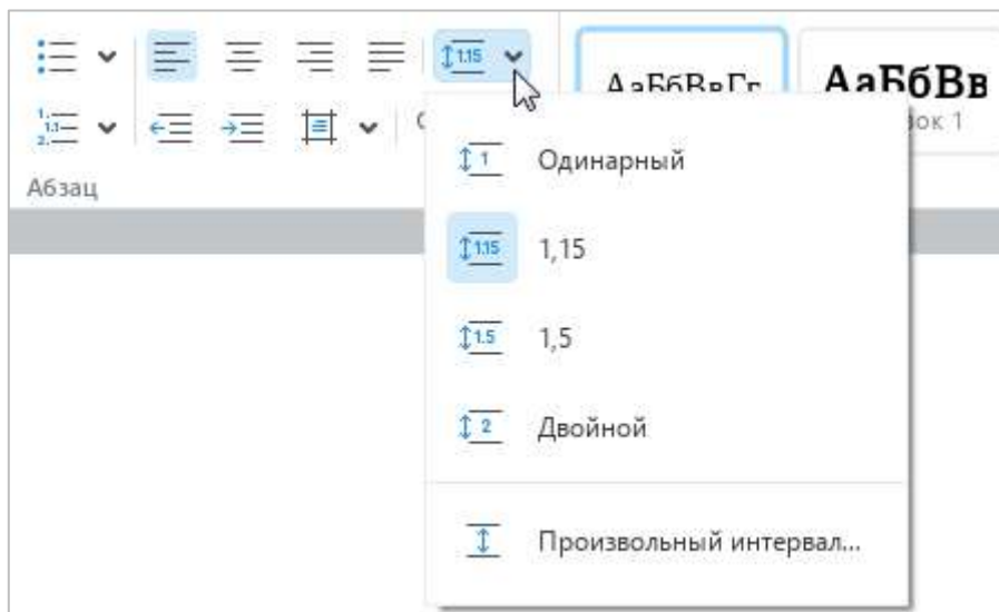
Рисунок 43 – Межстрочный интервал
