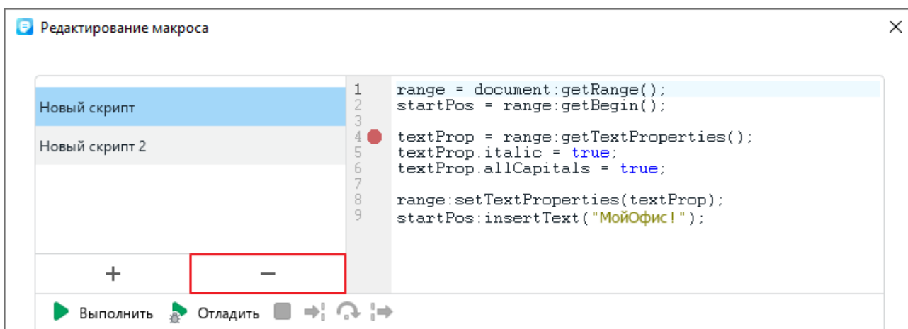
Рисунок 296 – Удаление макрокоманды
