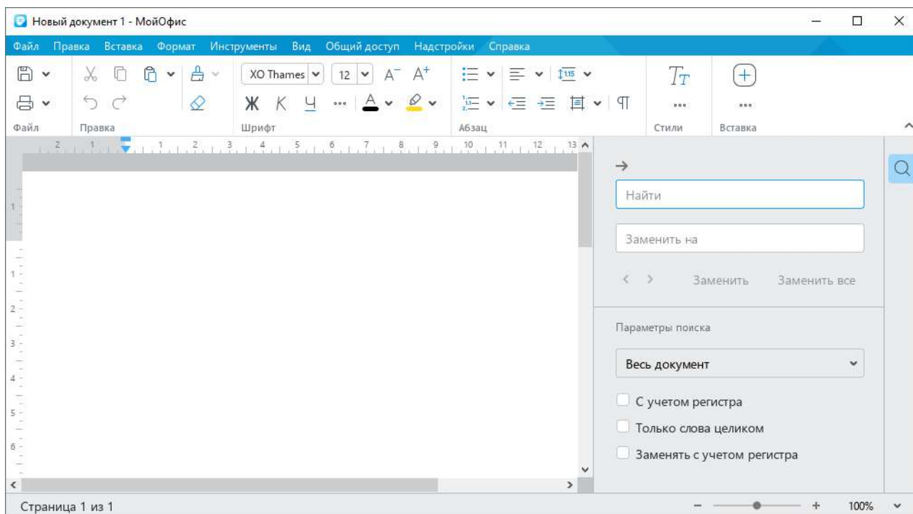
Рисунок 118 – Панель поиска
