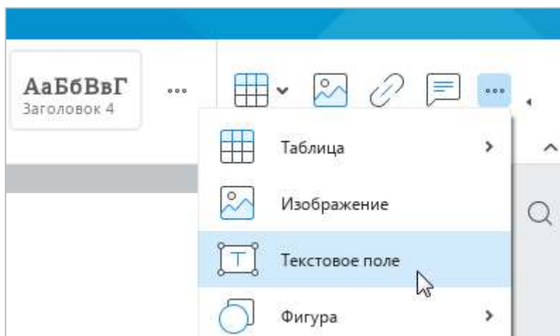
Рисунок 186 – Панель вставки
