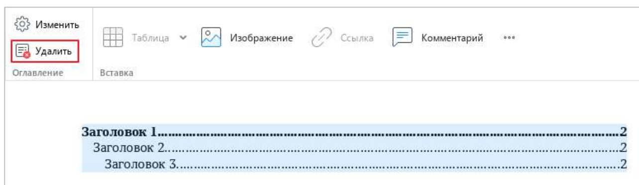
Рисунок 221 – Кнопка Удалить
