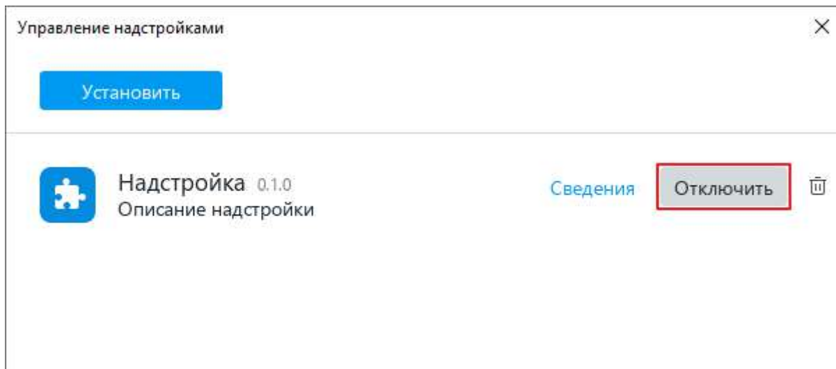
Рисунок 303 – Отключение надстройки
