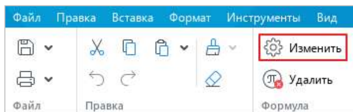
Рисунок 198 – Кнопка Изменить
