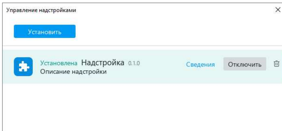
Рисунок 300 – Строка надстройки
