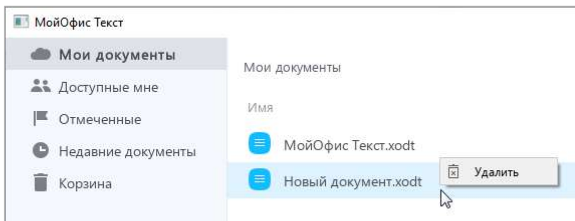
Рисунок 268 – Команда Удалить
