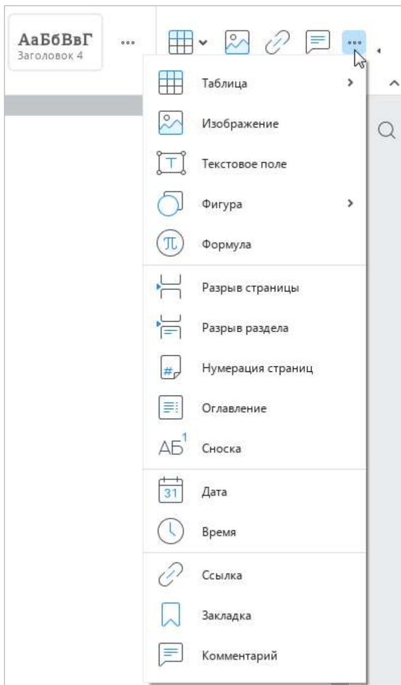
Рисунок 48 – Панель вставки
