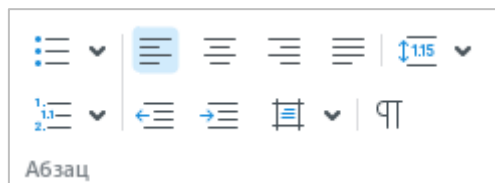
Рисунок 39 – Раздел Абзац
