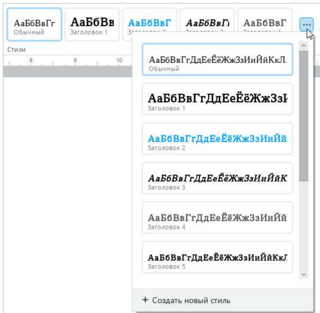
Рисунок 119 – Список стилей
