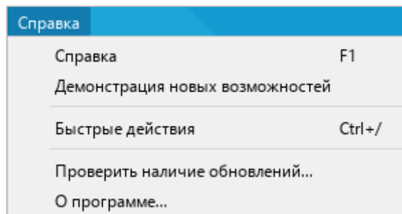
Рисунок 18 – Меню Справка
