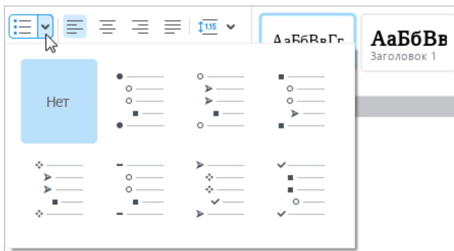
Рисунок 40 – Маркированный список
