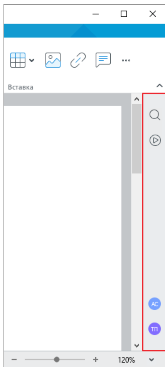
Рисунок 63 – Боковая панель
