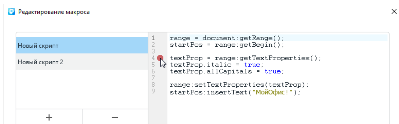
Рисунок 291 – Точка останова
