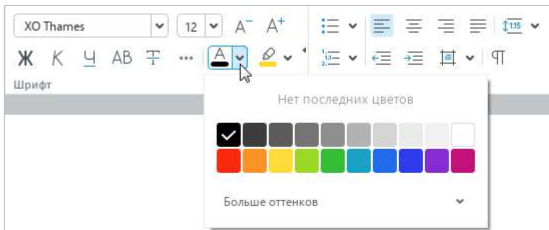
Рисунок 37 – Цвет текста
