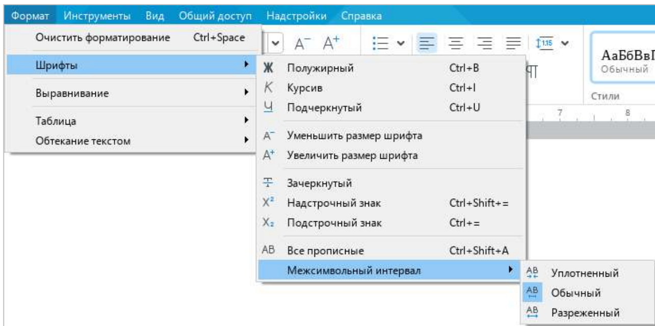
Рисунок 8 – Меню Формат
