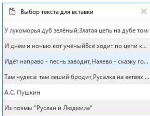
Рисунок 92 – Буфер обмена
