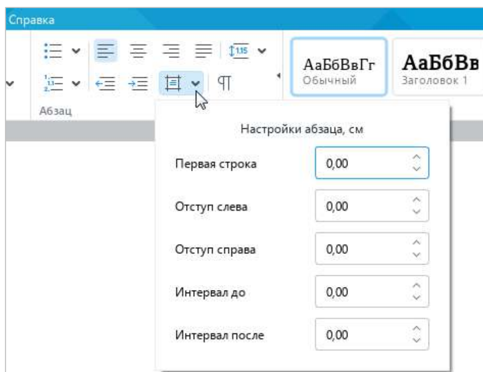
Рисунок 136 – Настройки абзаца
