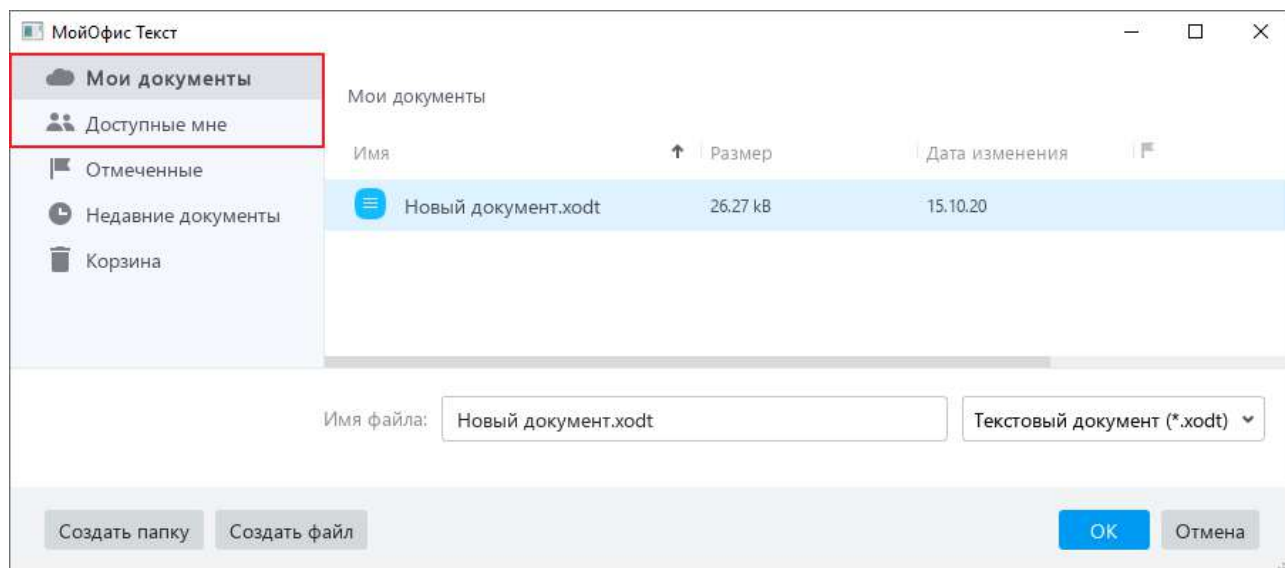
Рисунок 254 – Облачное хранилище
