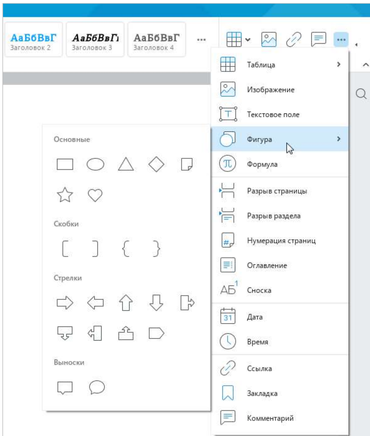
Рисунок 184 – Панель вставки
