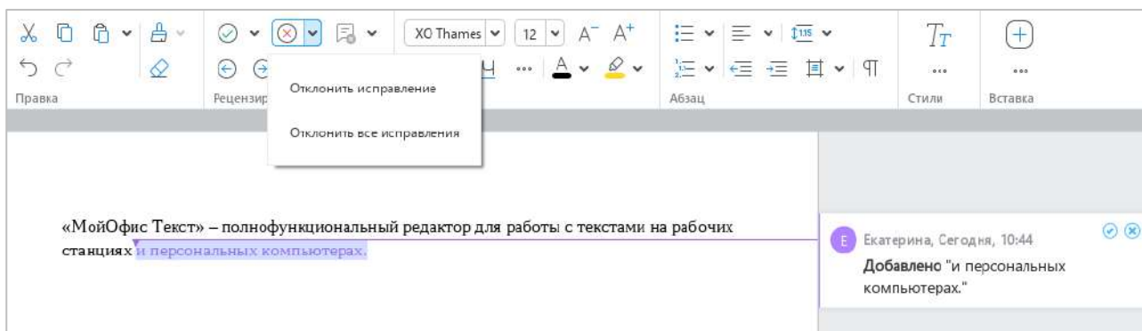
Рисунок 239 – Отклонение исправлений
