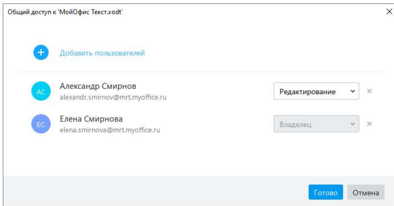
Рисунок 274 – Список пользователей
