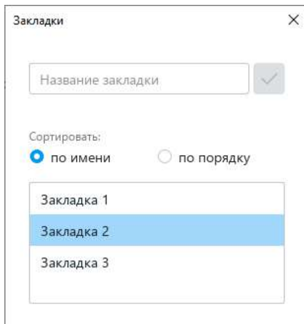
Рисунок 112 – Окно Закладки
