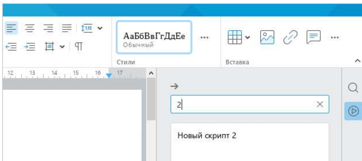
Рисунок 284 – Поиск макрокоманды
