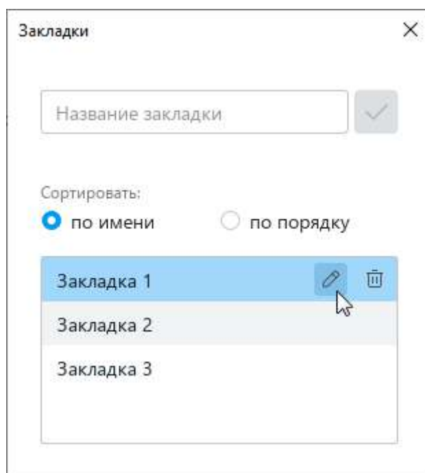
Рисунок 113 – Переименование закладки
