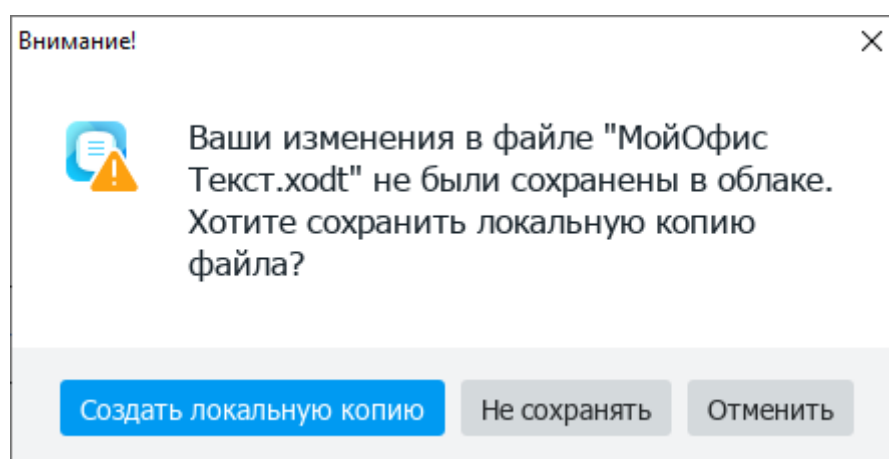
Рисунок 262 – Диалоговое окно
