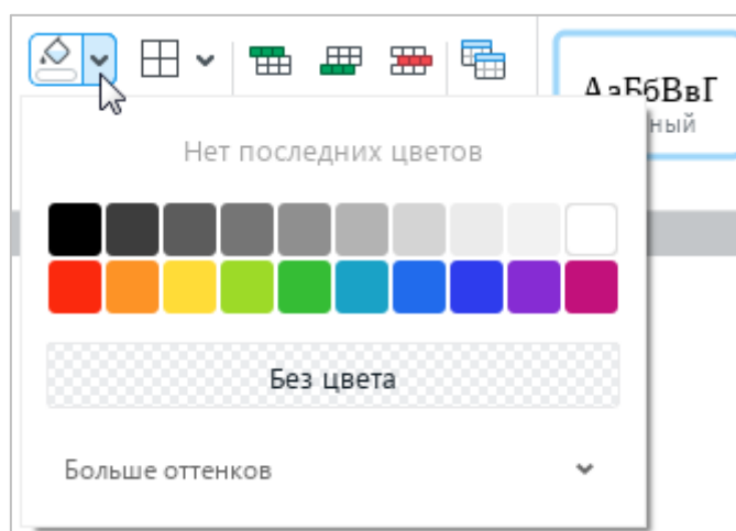
Рисунок 50 – Цвет заливки
