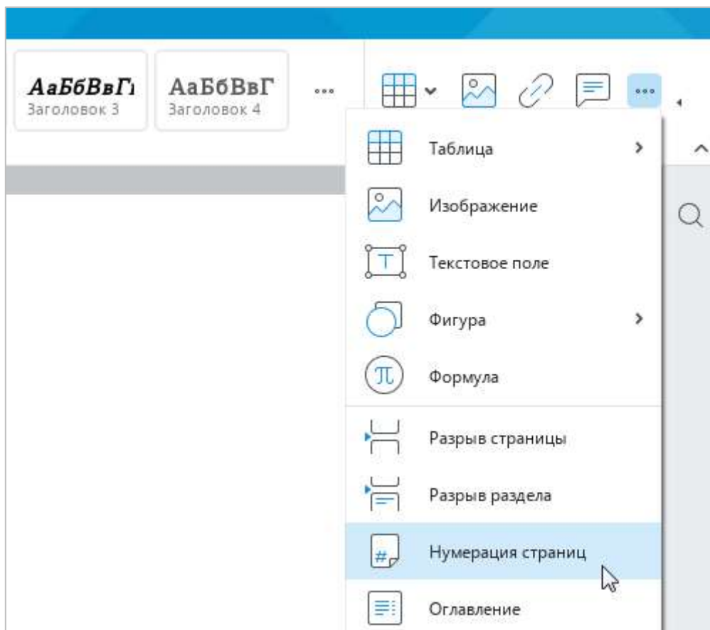
Рисунок 207 – Панель вставки
