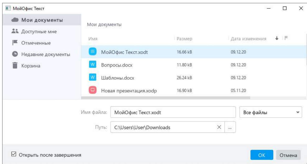
Рисунок 267 – Проводник
