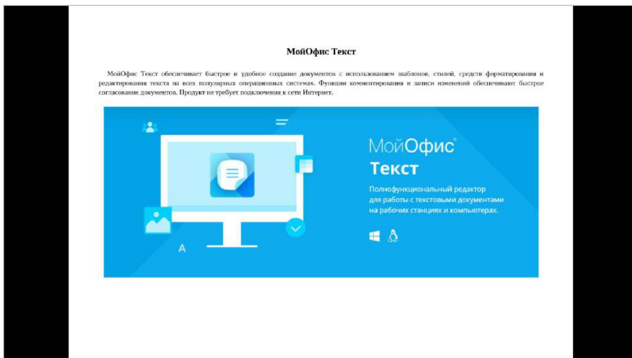
Рисунок 230 – Режим презентации
