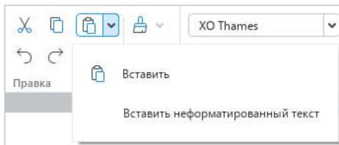
Рисунок 33 – Команды вставки
