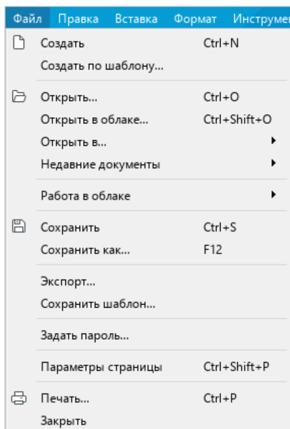
Рисунок 4 – Меню Файл
