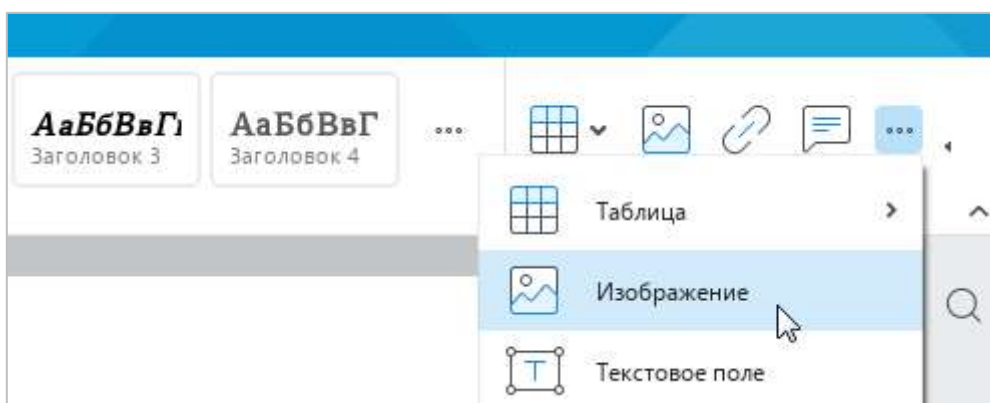
Рисунок 169 – Панель вставки
