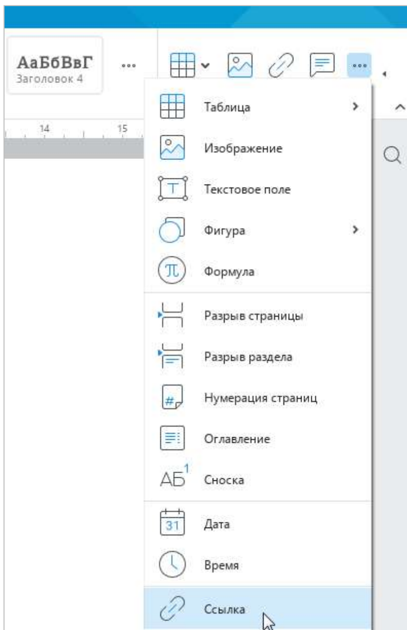
Рисунок 104 – Панель вставки
