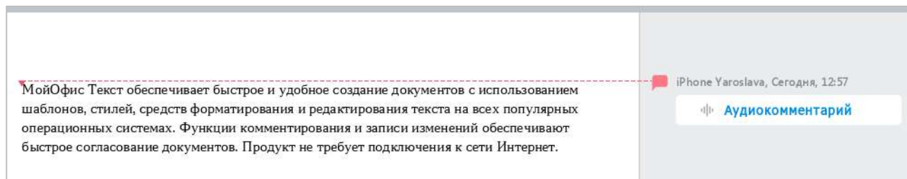
Рисунок 249 – Аудиокomentarий
