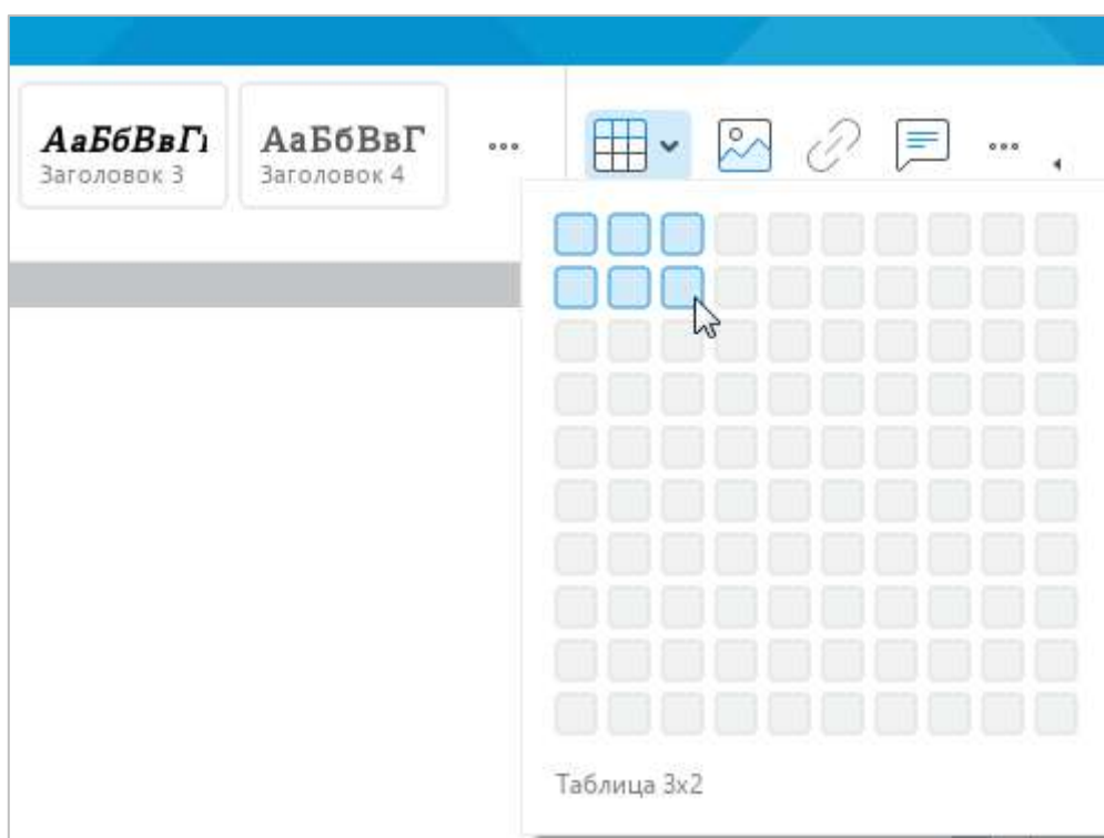
Рисунок 151 – Кнопка Таблица
