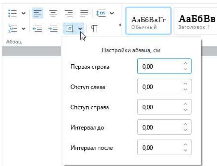
Рисунок 44 – Настройки абзаца
