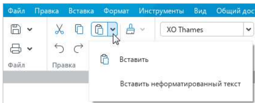
Рисунок 90 – Кнопка Вставить
