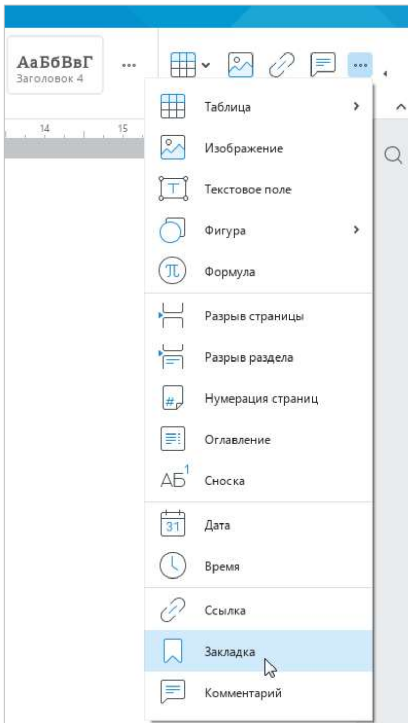
Рисунок 108 – Панель вставки
