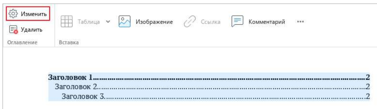
Рисунок 215 – Кнопка Изменить
