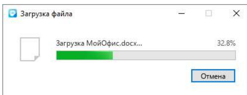
Рисунок 266 – Загрузка файла
