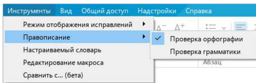
Рисунок 13 – Подменю Правописание
