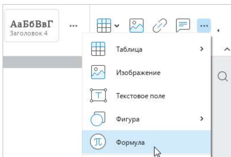
Рисунок 196 – Панель вставки
