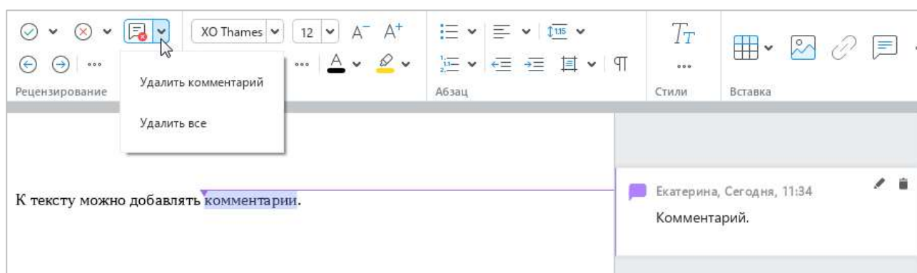
Рисунок 251 – Удаление комментария
