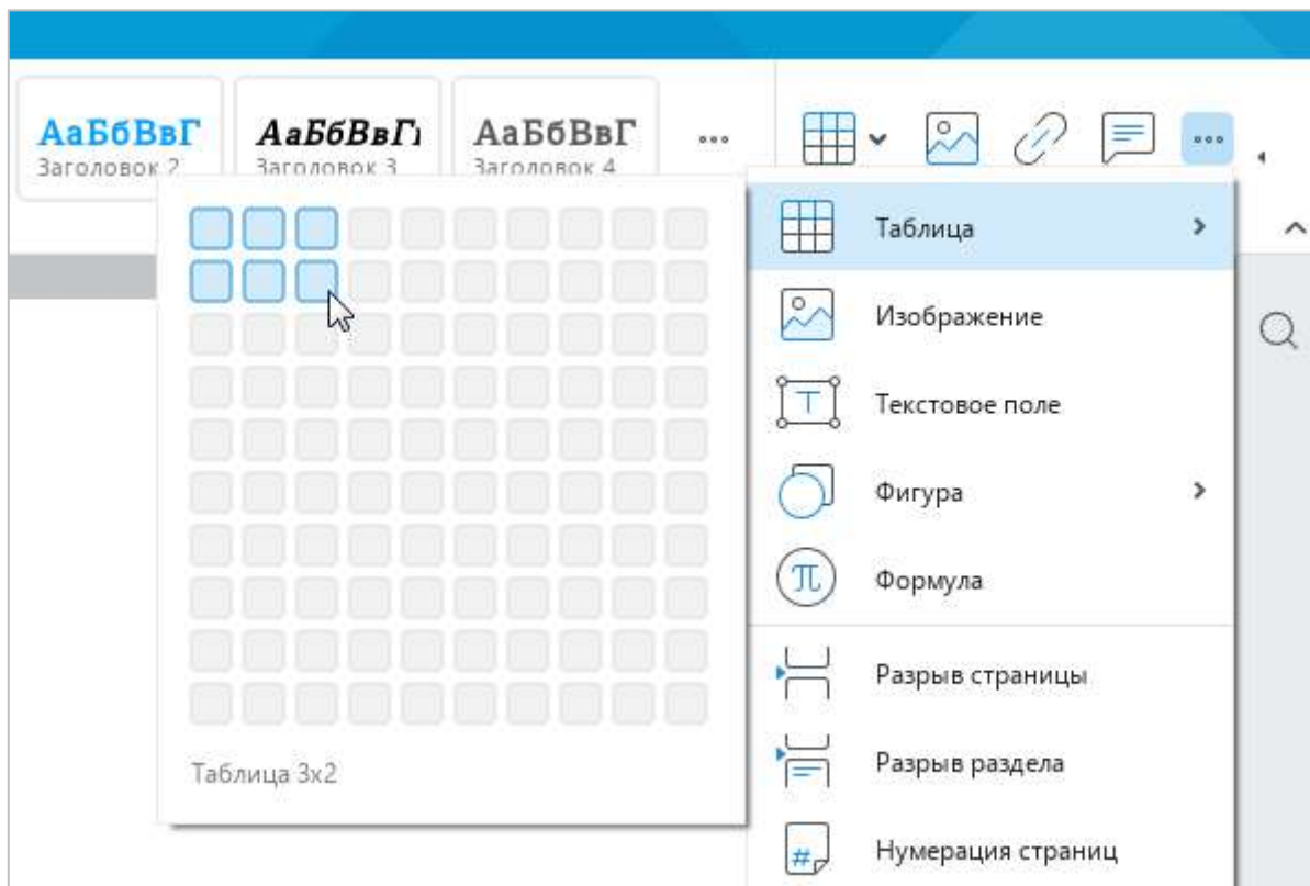
Рисунок 152 – Панель вставки
