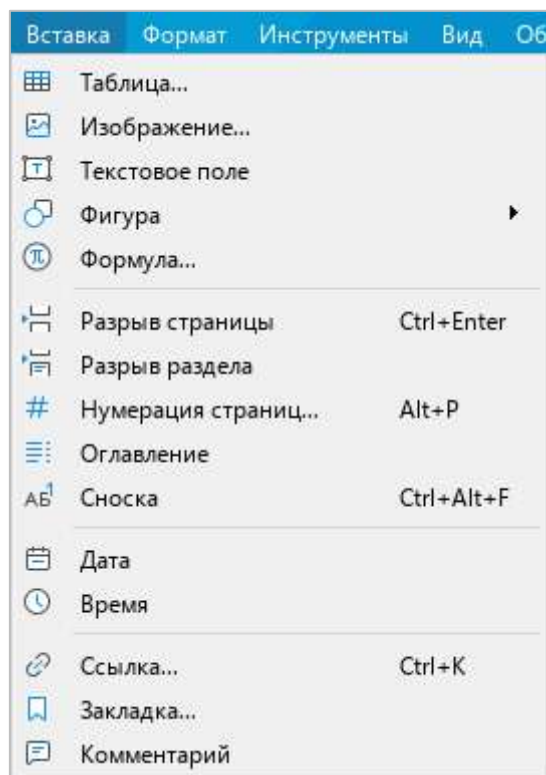
Рисунок 7 – Меню Вставка
