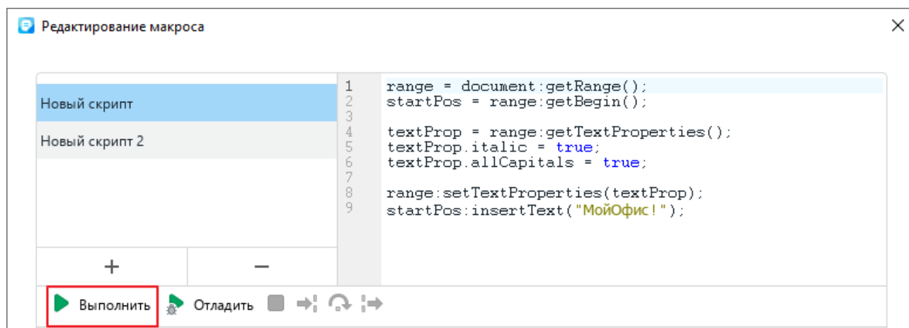
Рисунок 286 – Кнопка Выполнить
