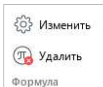
Рисунок 56 – Раздел Формула
