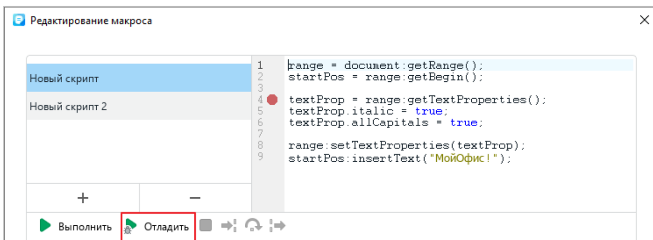
Рисунок 292 – Кнопка Отладить
