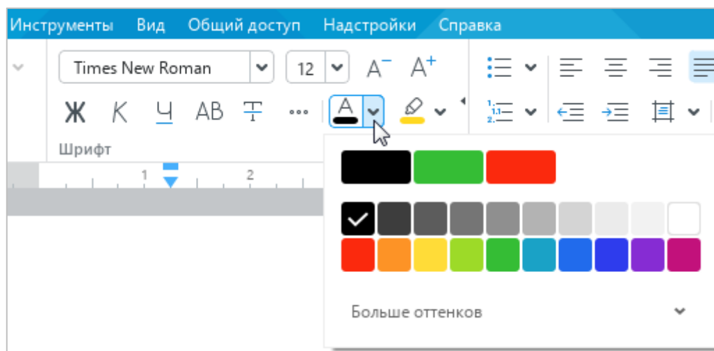
Рисунок 129 – Цвет текста
