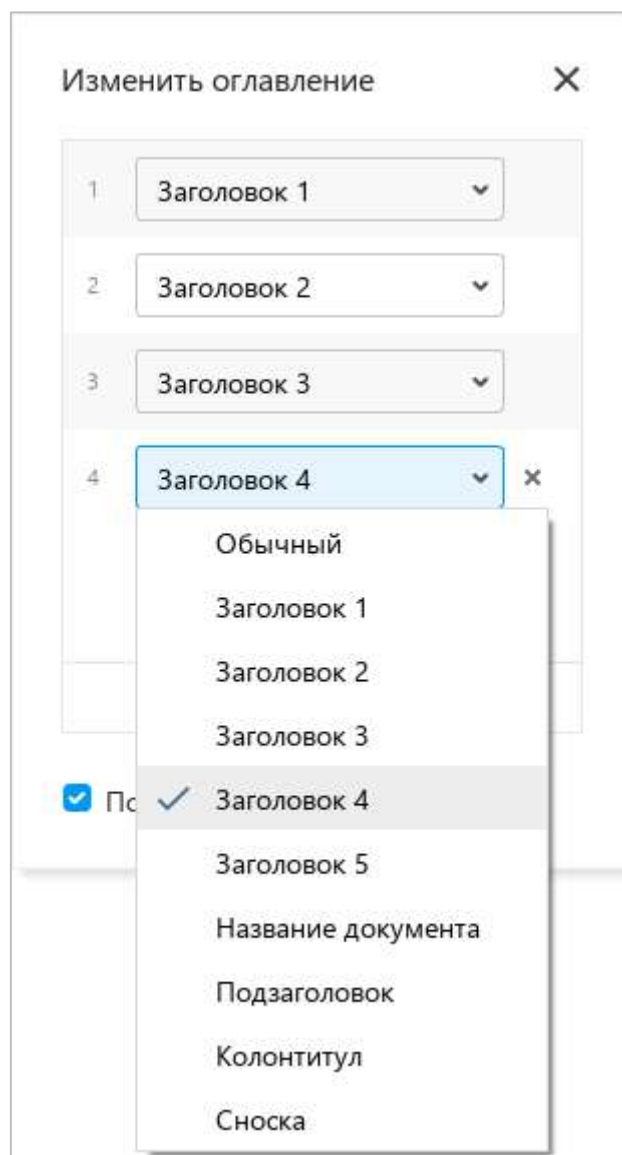
Рисунок 218 – Выбор стиля
