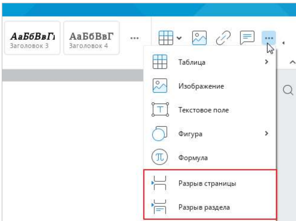
Рисунок 210 – Панель вставки
