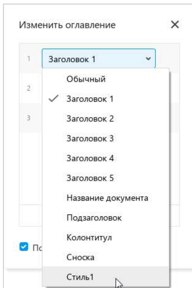
Рисунок 219 – Выбор стиля
