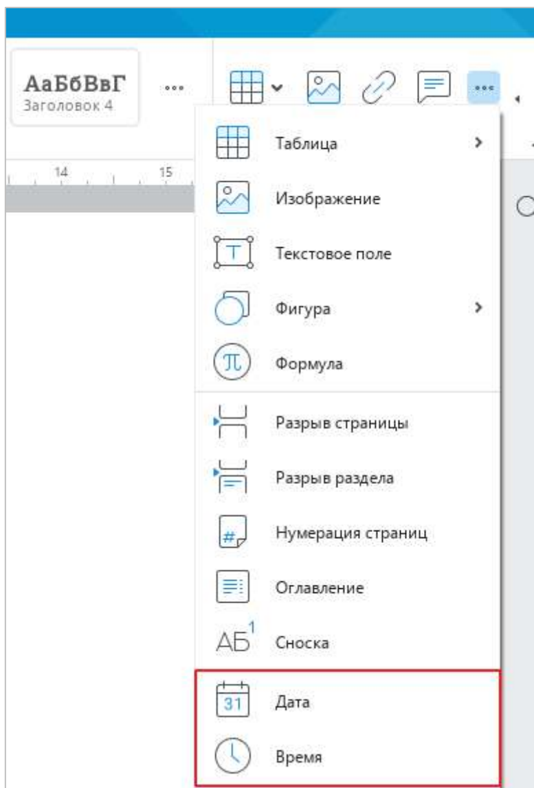
Рисунок 116 – Панель вставки
