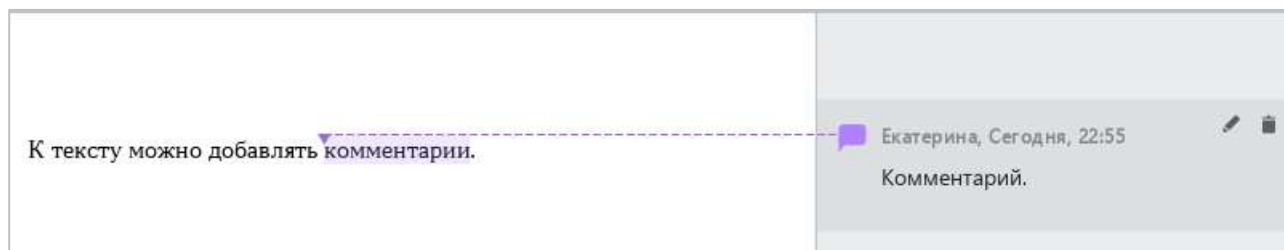
Рисунок 248 – Поле комментария
