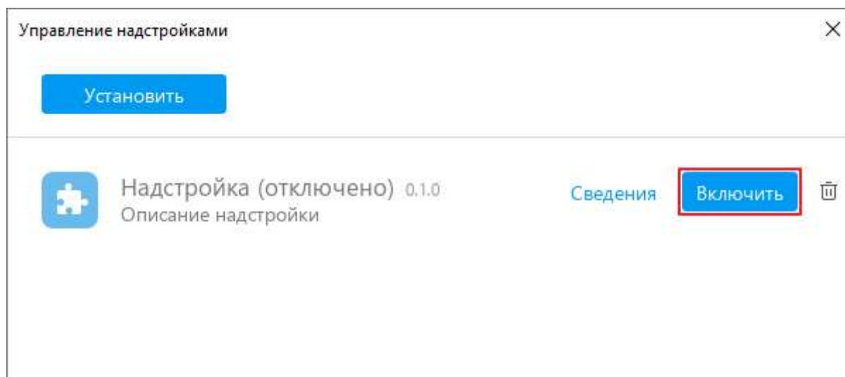
Рисунок 304 – Включение надстройки
