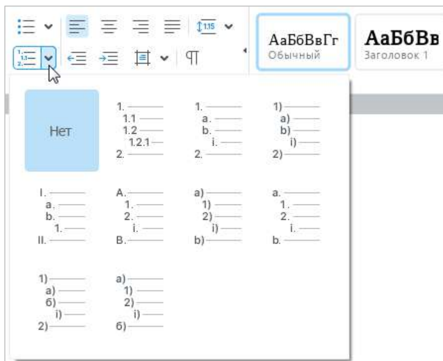
Рисунок 41 – Нумерованный список
