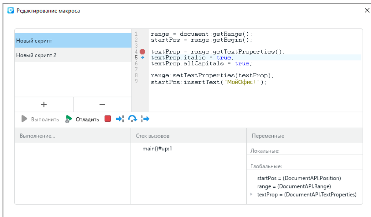
Рисунок 293 – Отладка макрокоманды
