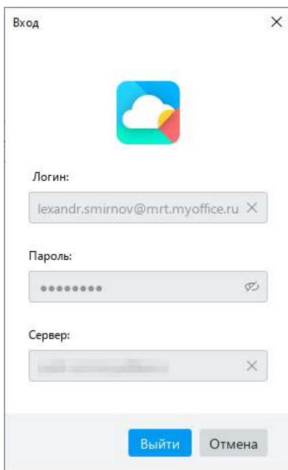
Рисунок 278 – Окно Вход
