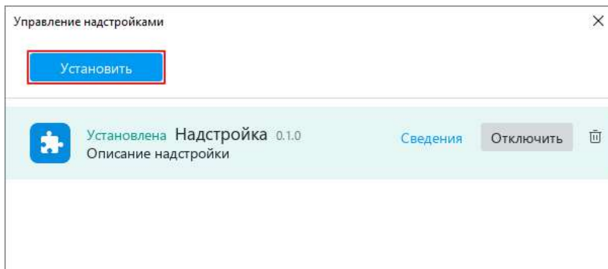
Рисунок 306 – Кнопка Установить
