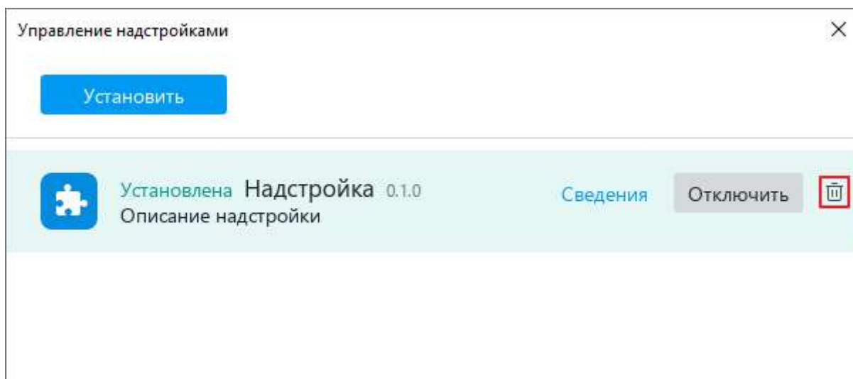
Рисунок 310 – Удаление надстройки
