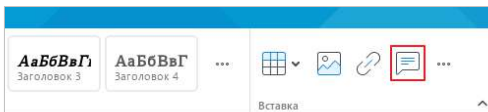
Рисунок 245 – Кнопка Комментарий
