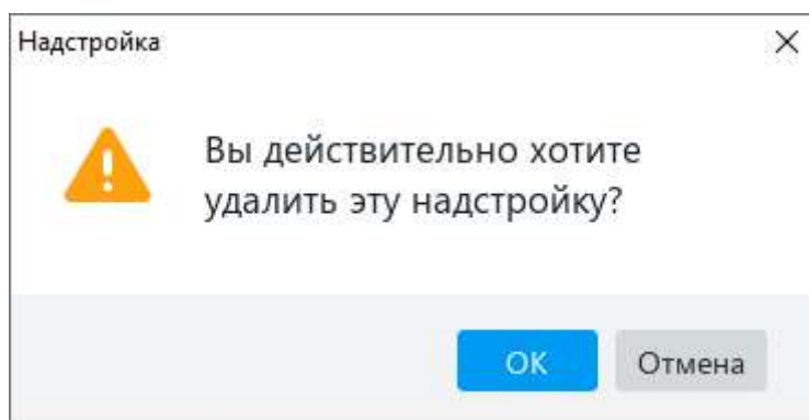
Рисунок 311 – Диалоговое окно
